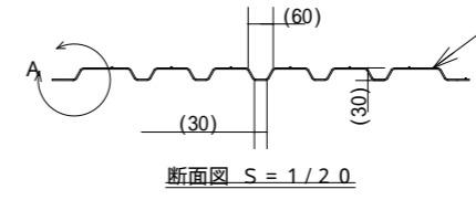
登はんヤシ繊維マット 詳細図 S=1/20
